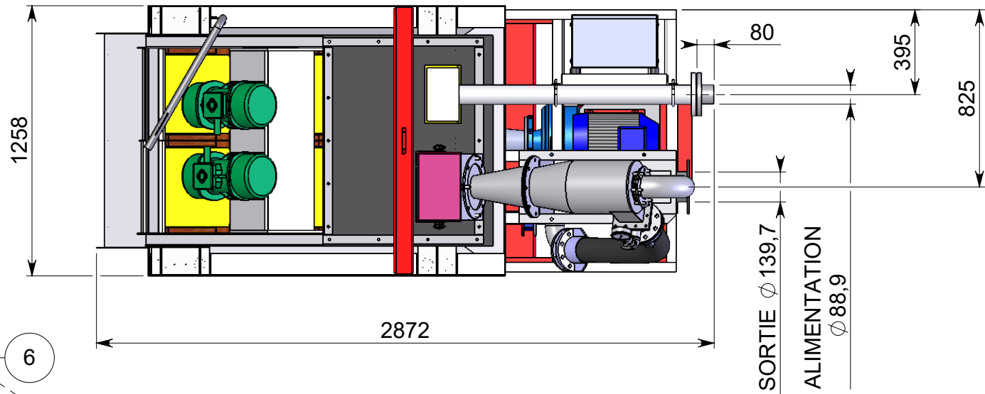
Ø 200 ALIMENTATION Bride DN80 PN10 Ø ext.200 ép.22 8 trous Ø 18 sur Ø 160 Trous hors axe ou adaptateur tube lisse Øext.88.9
